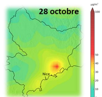
Maximum journalier en particules le 28/10/2017 visualisez la carte régionale
